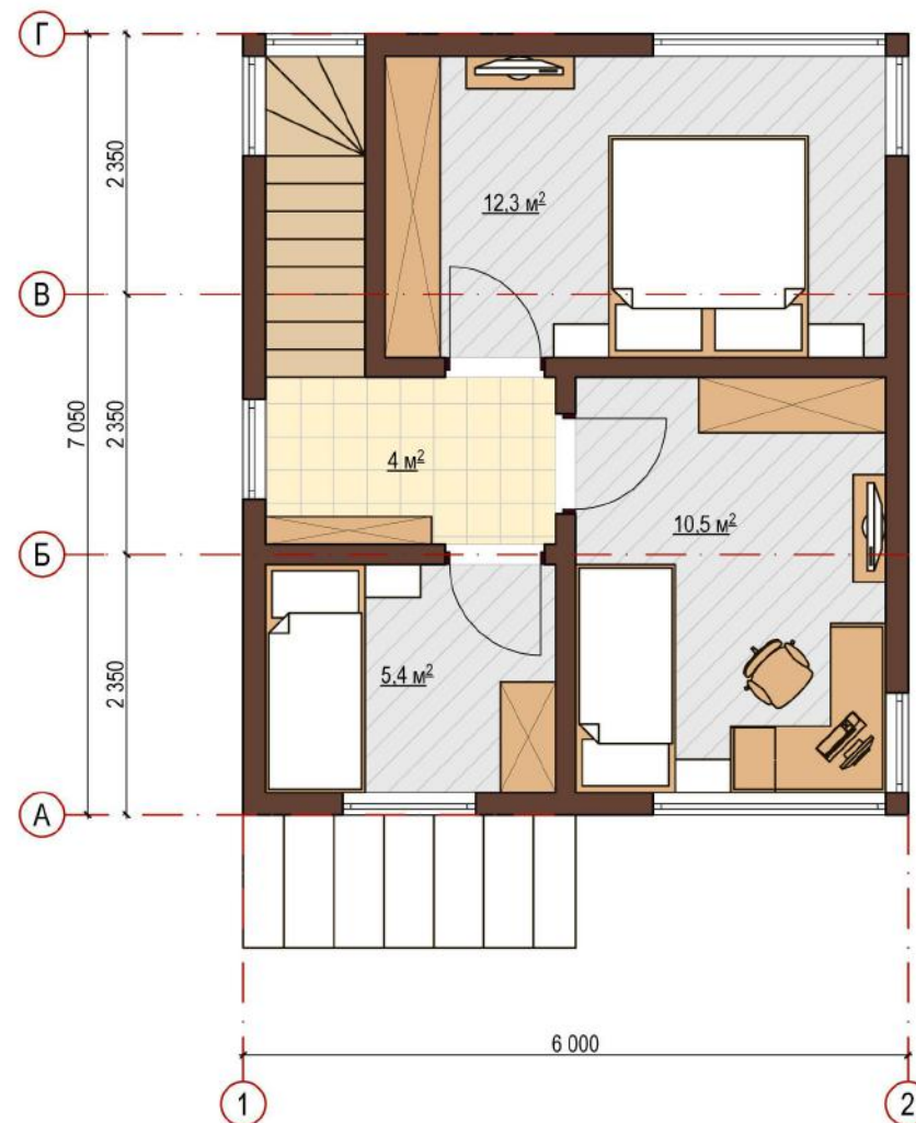
План 2-го этажа
